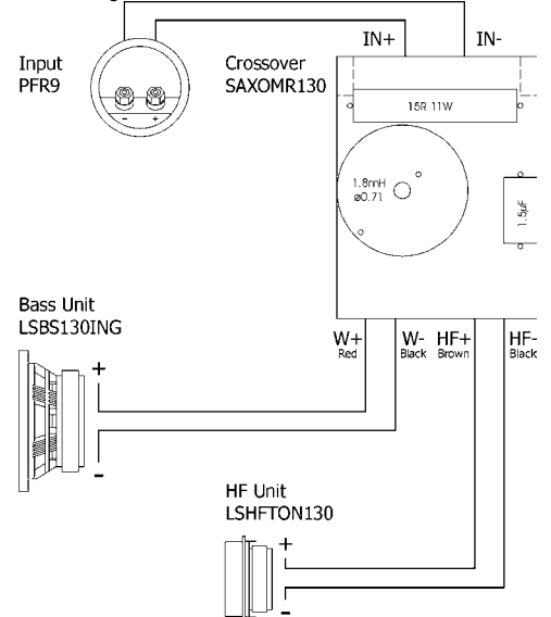
Verdrahtungsschema
