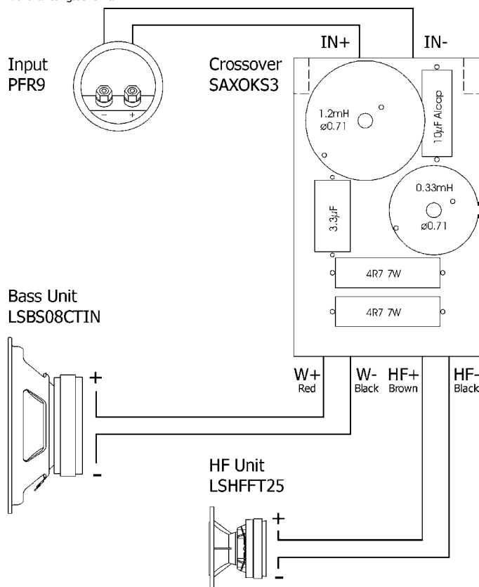
Verdrahtungsschema
